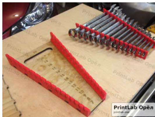
Органайзер гаечных ключей
