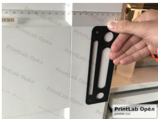
Шаблон установки ручки
