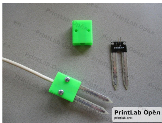
Держатель датчика влажности почвы
